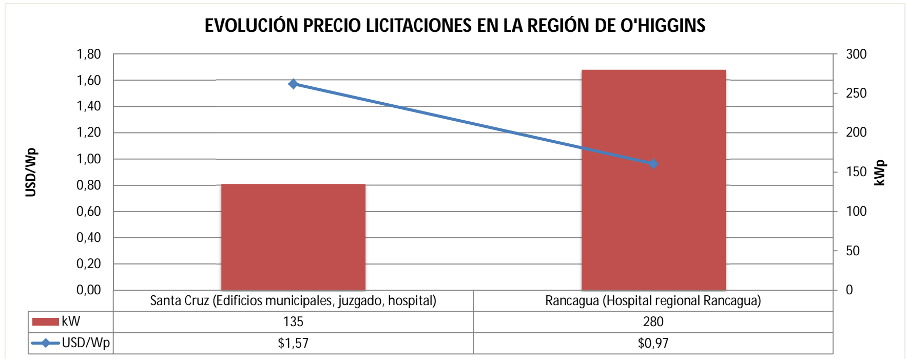
Gráfico 18 – Precio y potencia de las licitaciones adjudicadas en la región de O'Higgins
