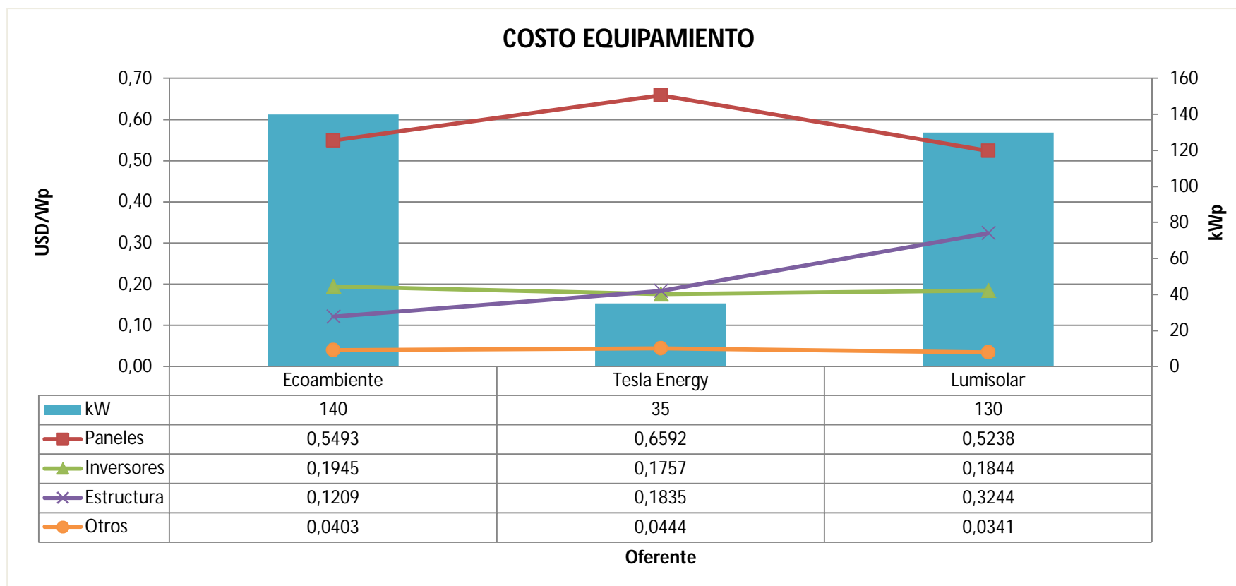
Gráfico 13 – Estructura de costos de equipamiento licitaciones en la región de Coquimbo
