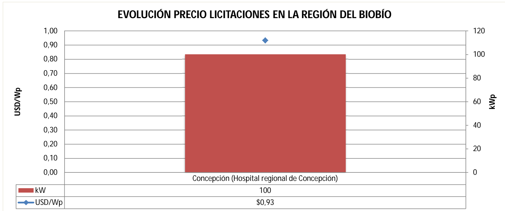
Gráfico 22 - Precio y potencia de las licitaciones adjudicadas en la región del Biobío
