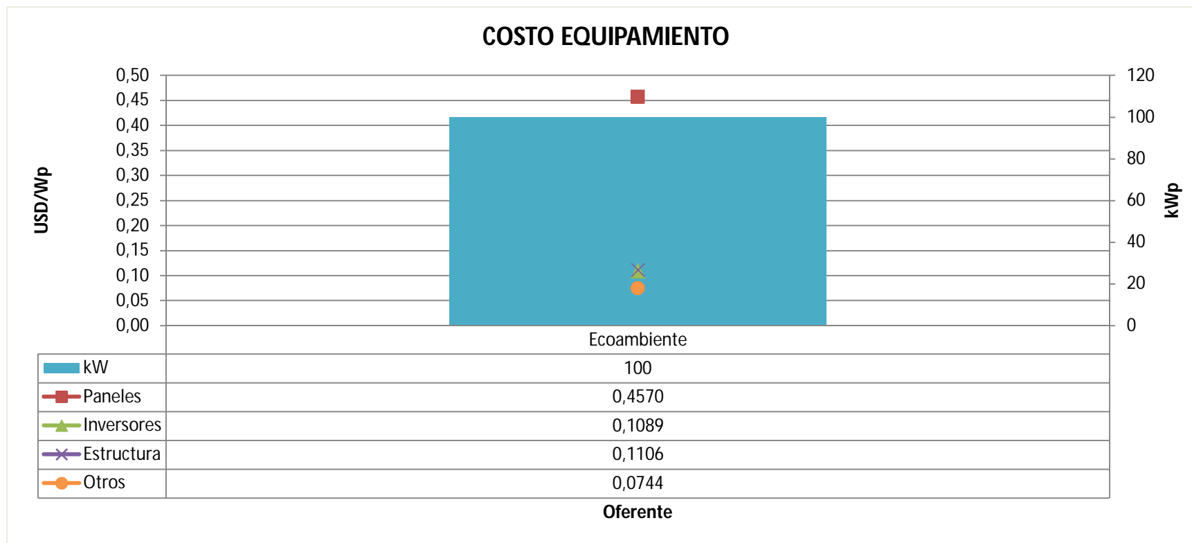
Gráfico 23 – Estructura de costos de equipamiento licitaciones en la región del Biobío
