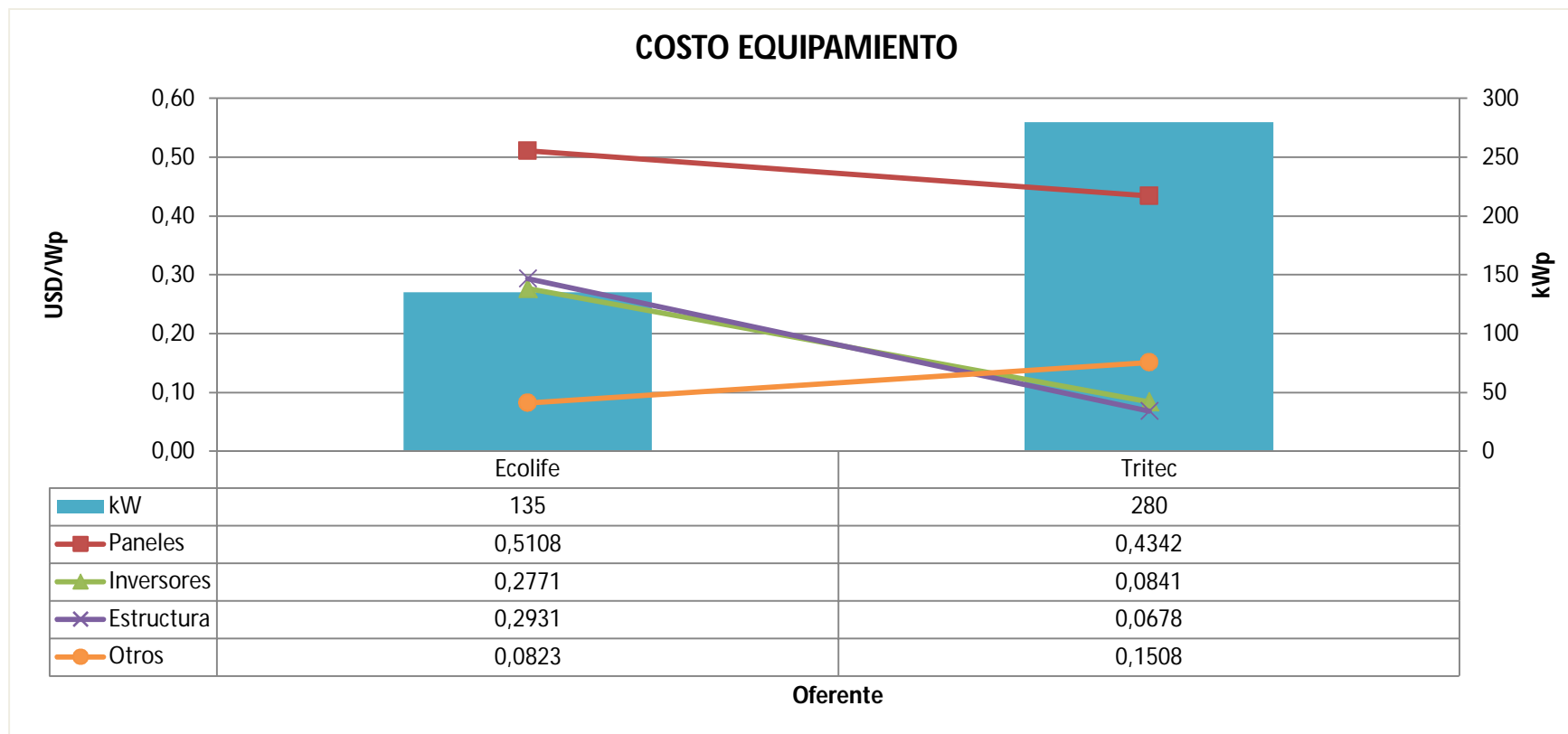
Gráfico 19 – Estructura de costos de equipamiento licitaciones en la región de O'Higgins
