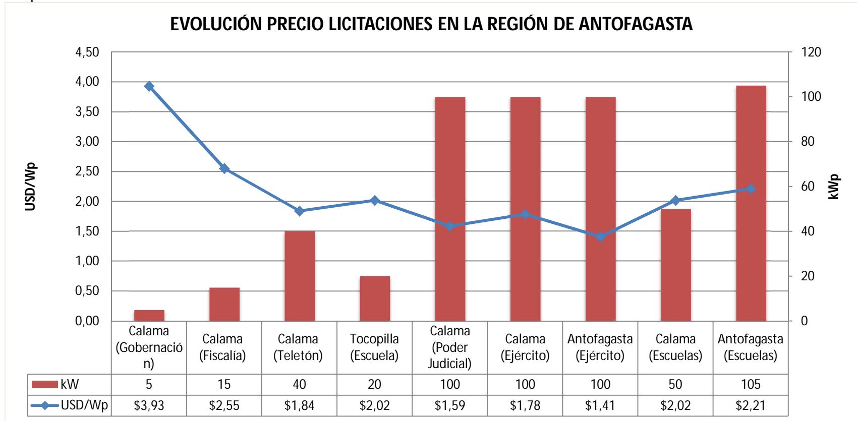
Gráfico 8 – Precio y potencia de las licitaciones adjudicadas en la región de Antofagasta
