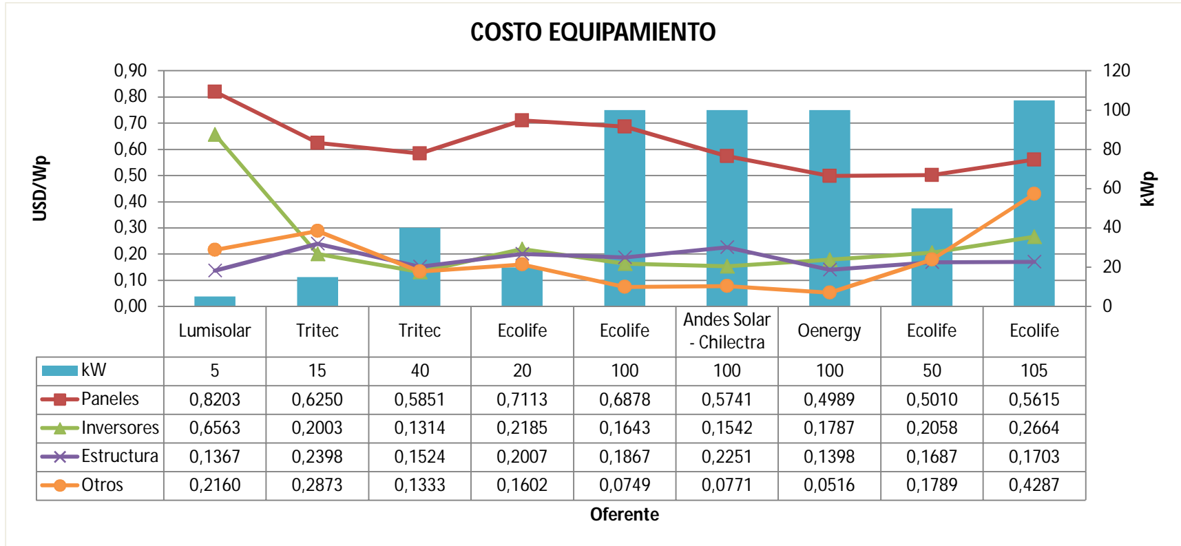
Gráfico 9 – Estructura de costos de equipamiento licitaciones en la región de Antofagasta
