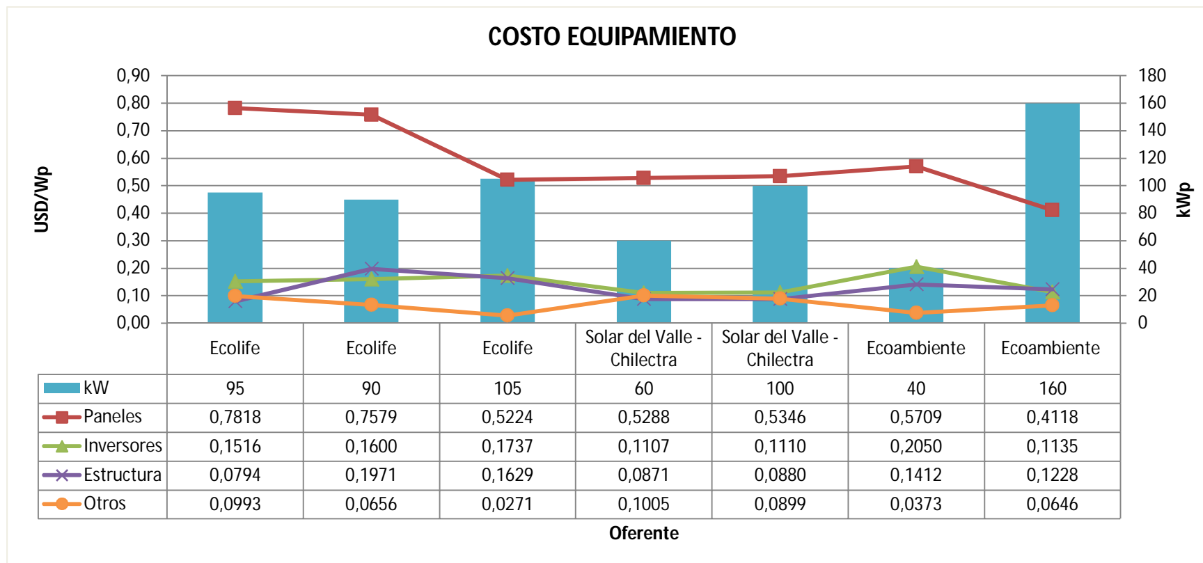
Gráfico 21 – Estructura de costos de equipamiento licitaciones en la región del Maule
