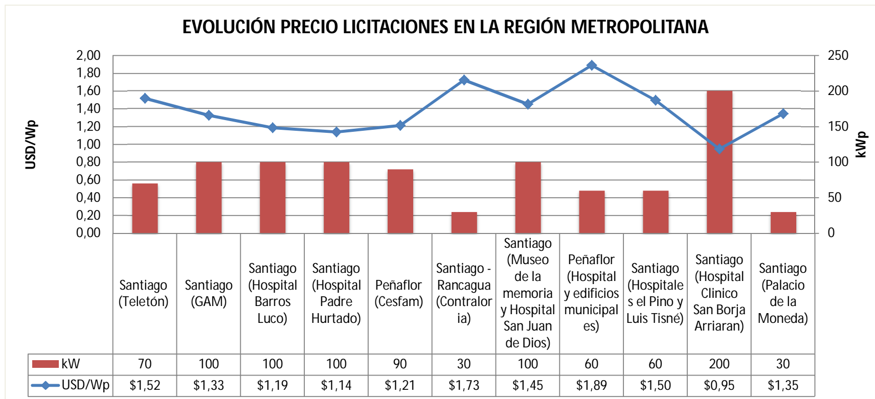
Gráfico 16 – Precio y potencia de las licitaciones adjudicadas en la región de Metropolitana
