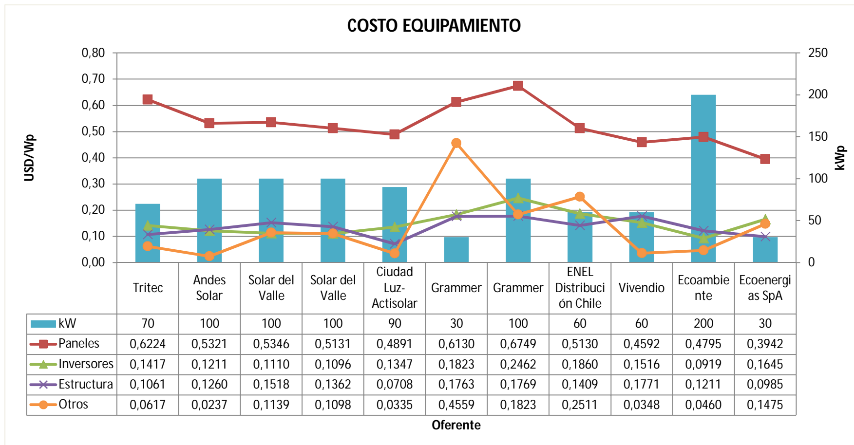
Gráfico 17 – Estructura de costos de equipamiento licitaciones en la región Metropolitana
