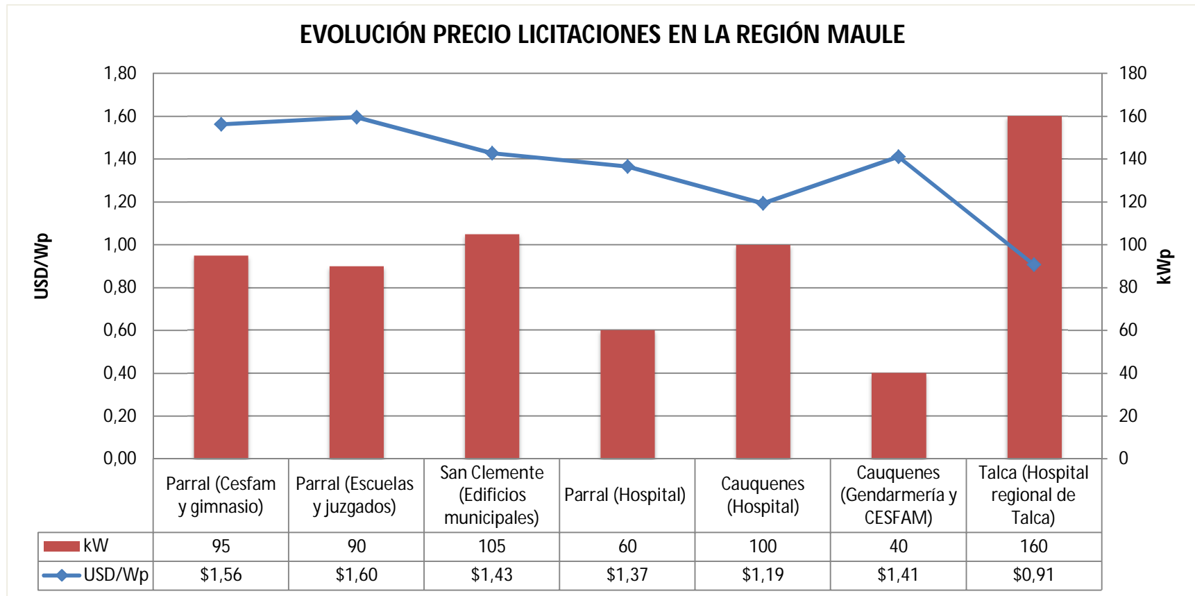
Gráfico 20 – Precio y potencia de las licitaciones adjudicadas en la región del Maule
