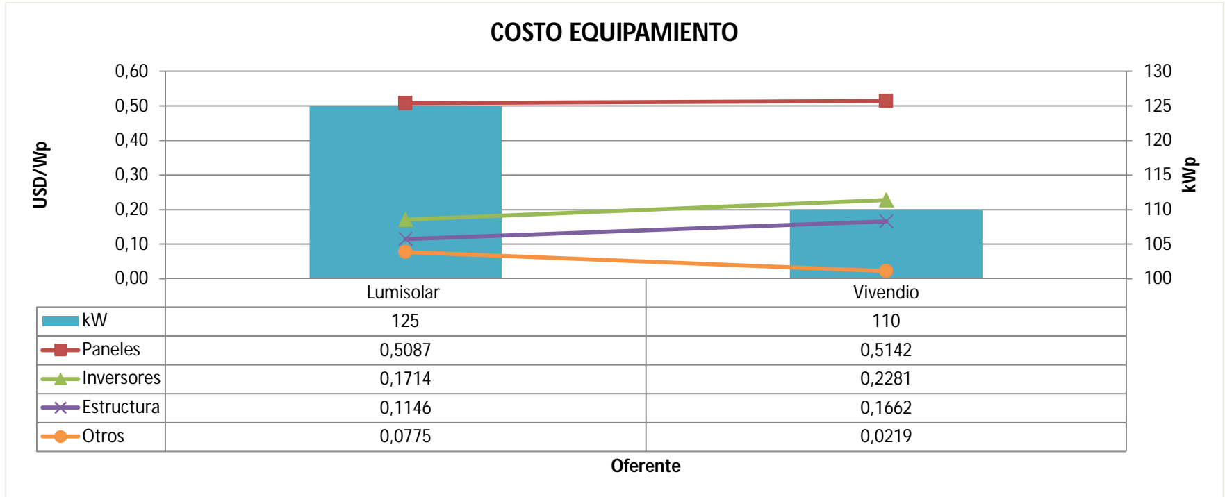
Gráfico 15 – Estructura de costos de equipamiento licitaciones en la región de Valparaíso
