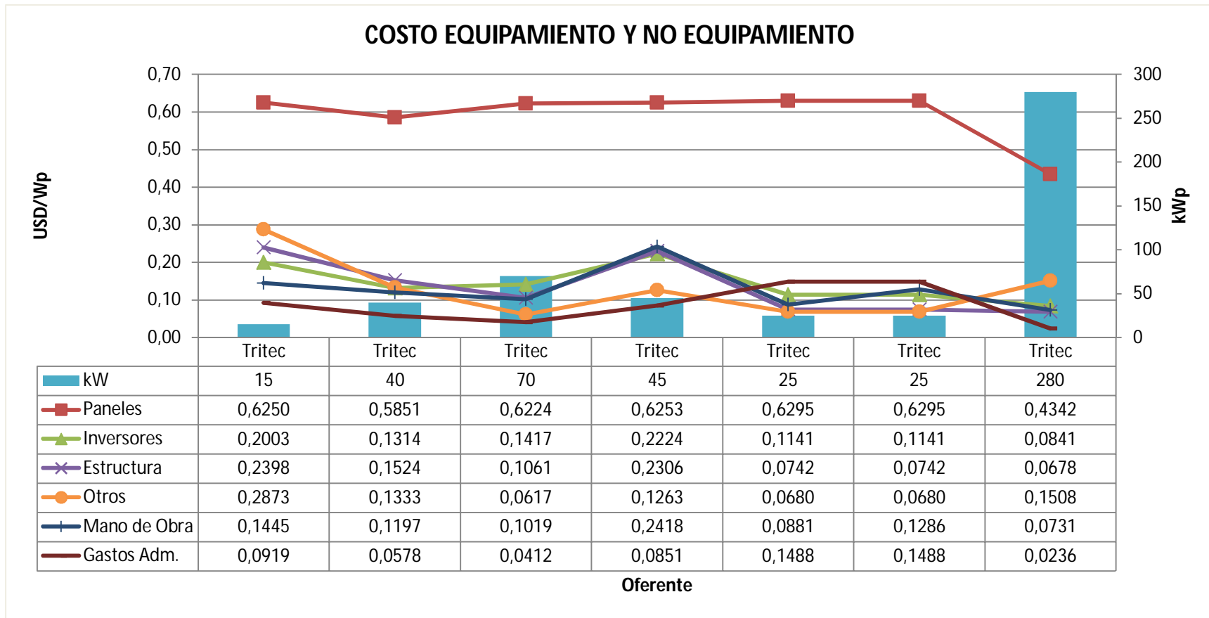
Gráfico 32 – Estructura de costos licitaciones adjudicadas por Tritec
