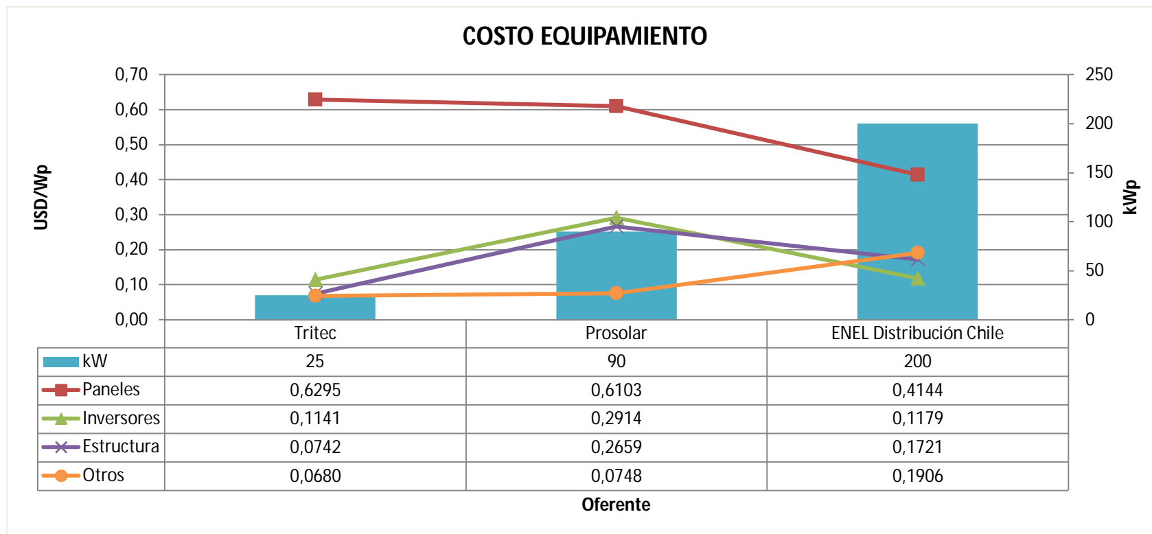
Gráfico 7 – Estructura de costos de equipamiento licitaciones en la región de Tarapacá
