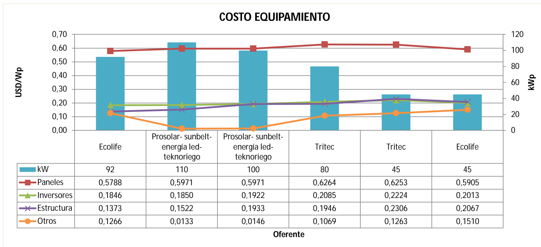
Gráfico 11 – Estructura de costos de equipamiento licitaciones en la región de Atacama
