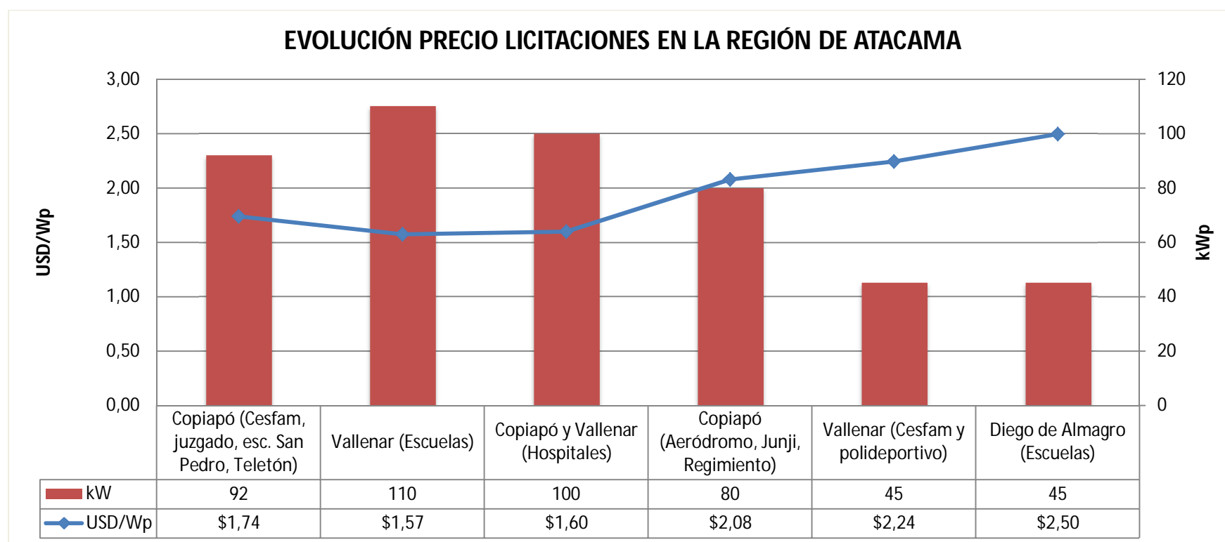
Gráfico 10 – Precio y potencia de las licitaciones adjudicadas en la región de Atacama
