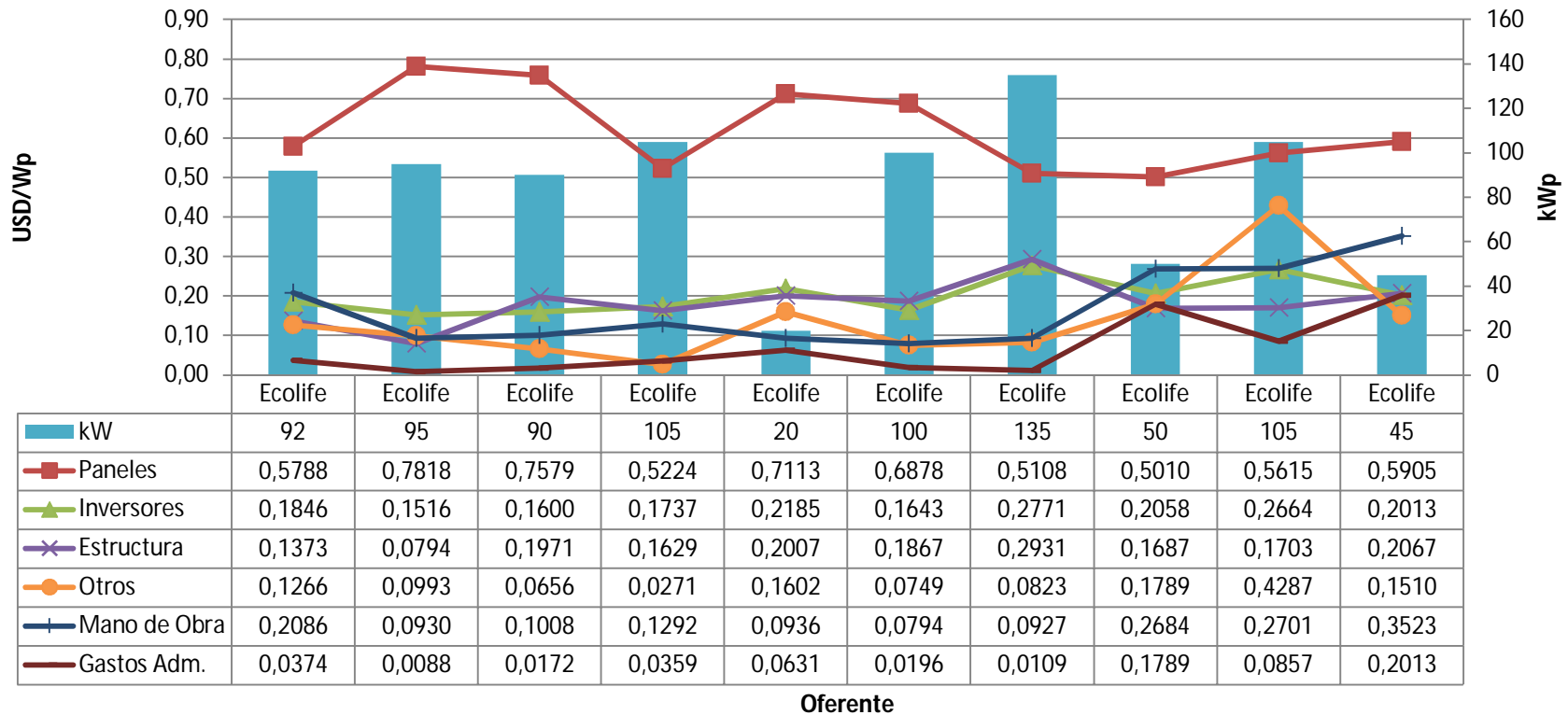
Gráfico 28 – Estructura de costos licitaciones adjudicadas por Ecolife
