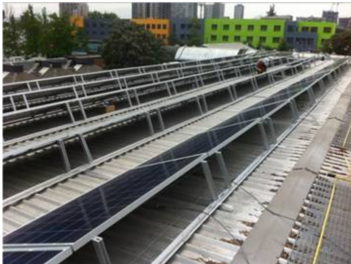
Ilustración. Estructura de anclaje típica para módulos fotovoltaicos inclinados sobre cubierta. Foto proyecto Teletón Santiago, Programa Techos Solares Públicos
