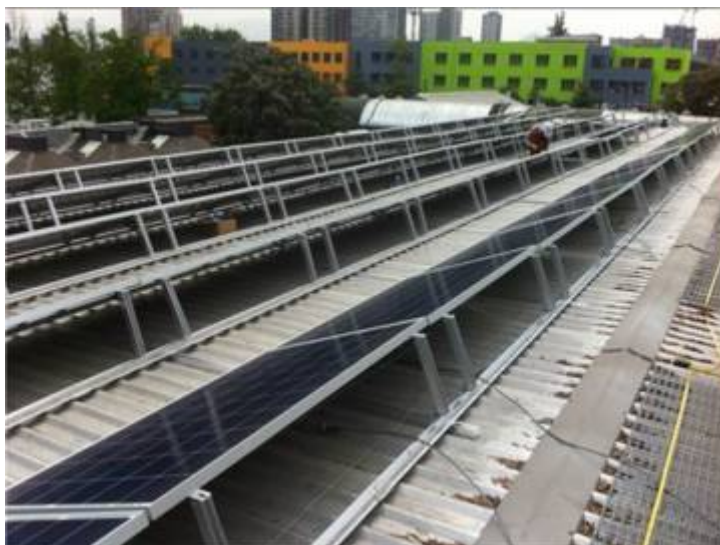
Ilustración 1. Estructura de anclaje típica para módulos fotovoltaicos inclinados sobre cubierta. Foto proyecto Teletón Santiago, Programa Techos Solares Públicos
