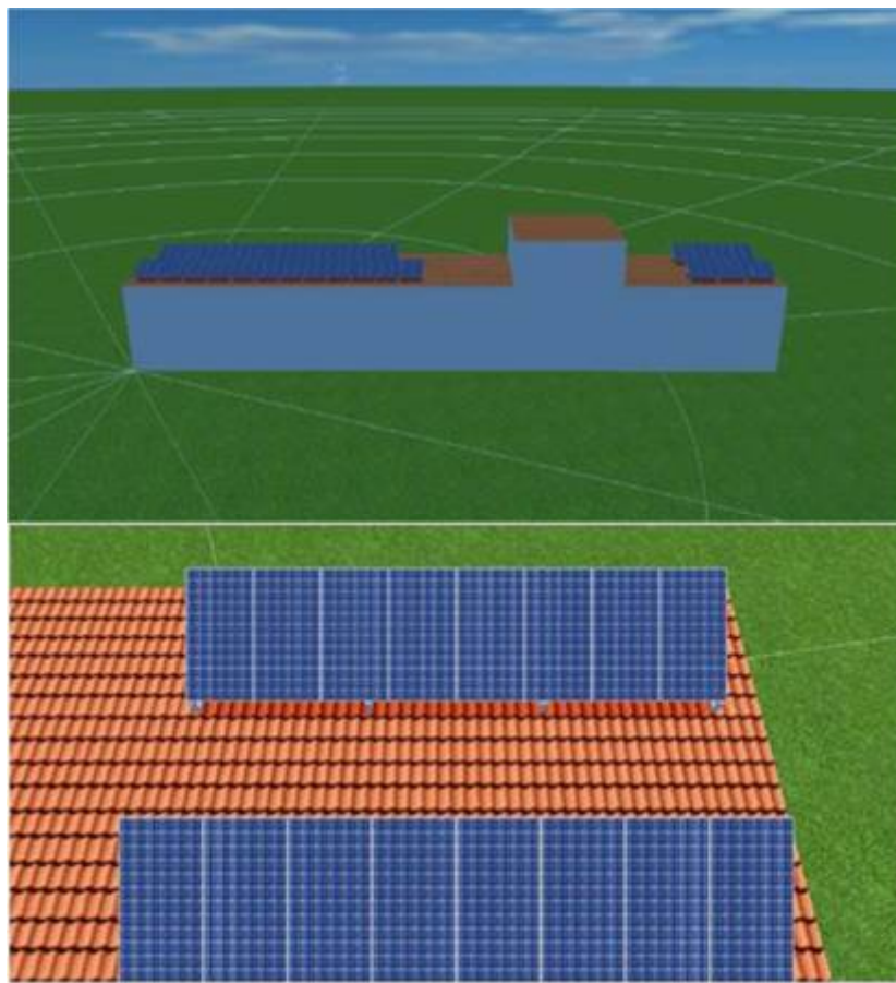
Figura: Planificación 3D de Copia 1 de Edificio 01-Superficie del tejado norte
