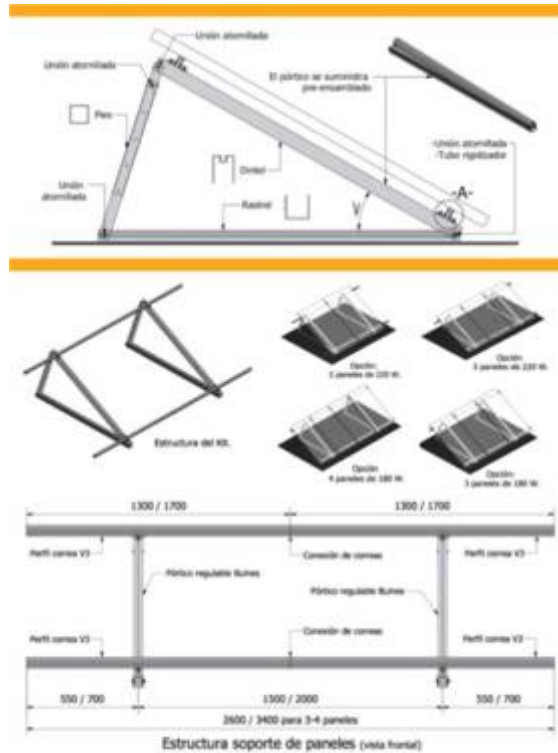
Ilustración 2. Estructura tipo inclinada sobre techo plano
