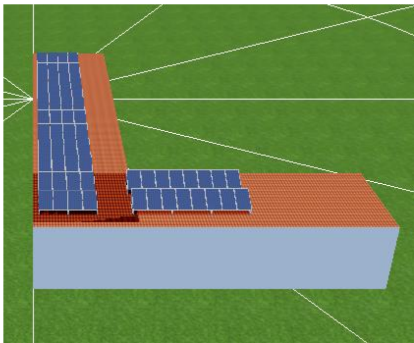
Ilustración – Vista simulación Orientación Norte
