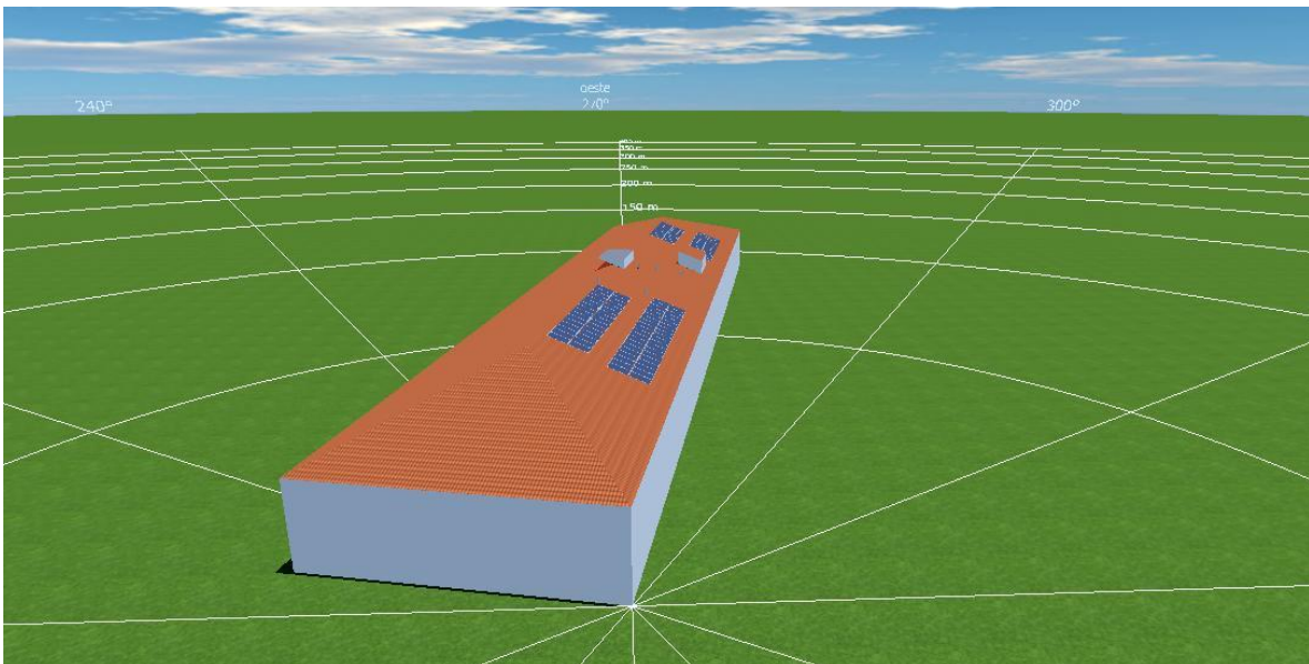
Ilustración – Vista simulación orientación este
