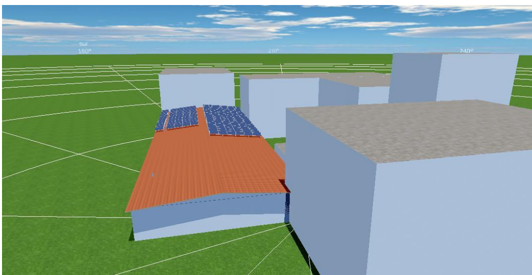
Ilustración – Vista simulación orientación norte
