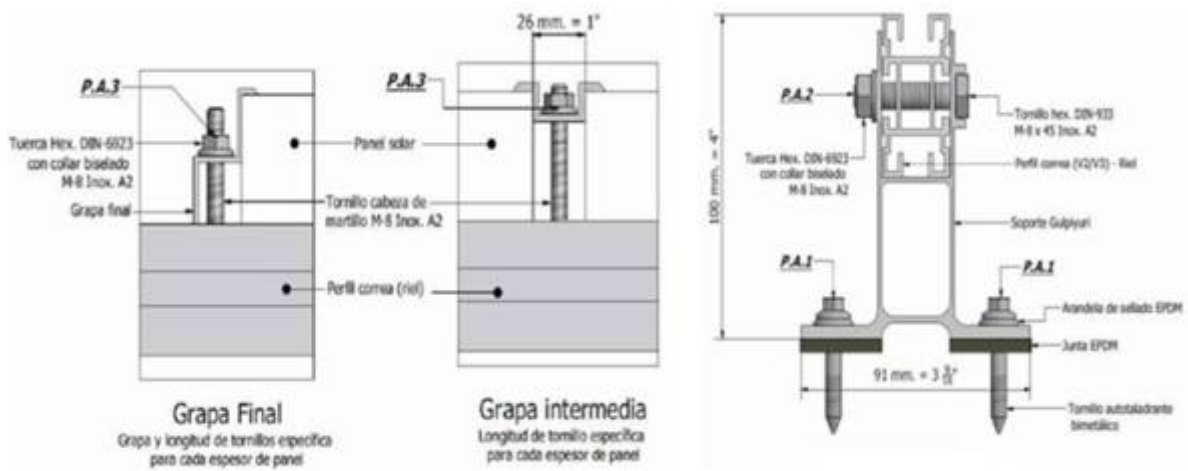
Ilustración. Sistema de montaje paralelo a cubierta
