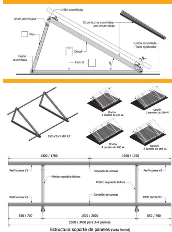
Ilustración 1. Estructura tipo inclinada sobre techo plano
