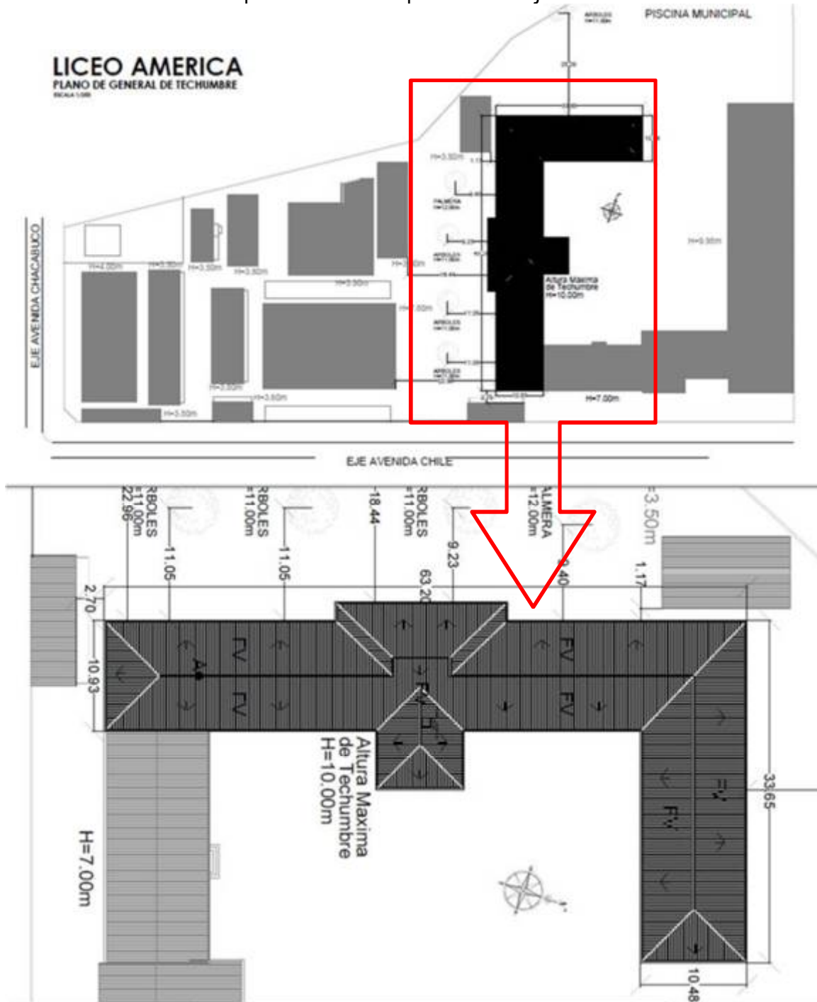
Ilustración – Esquema cubierta techo seleccionado
