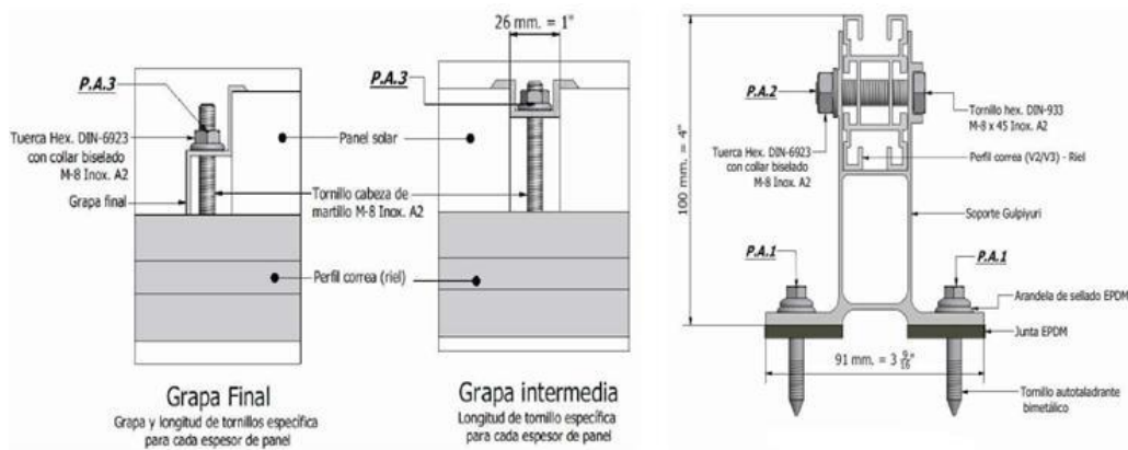
Ilustración 3. Sistema de montaje
