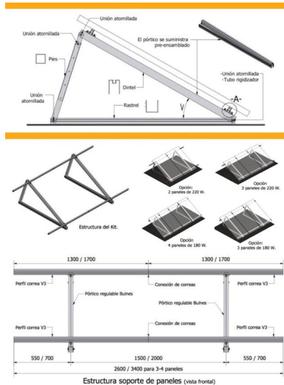
Ilustración 2. Estructura tipo inclinada sobre techo plano
