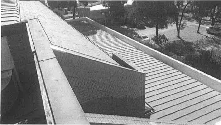
4.3 Techo de 2 aguas, edificio 2
