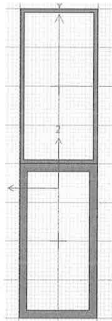
Ilustración – Refuerzo propuesto en vigas de los ejes 14', 15' y las vigas transversales, compuesto por un perfil cajón 4 x 0,89 existente y un perfil cajón 4 x 1,68 soldados entre si. Ejes según planos de cálculo del edificio principal.
