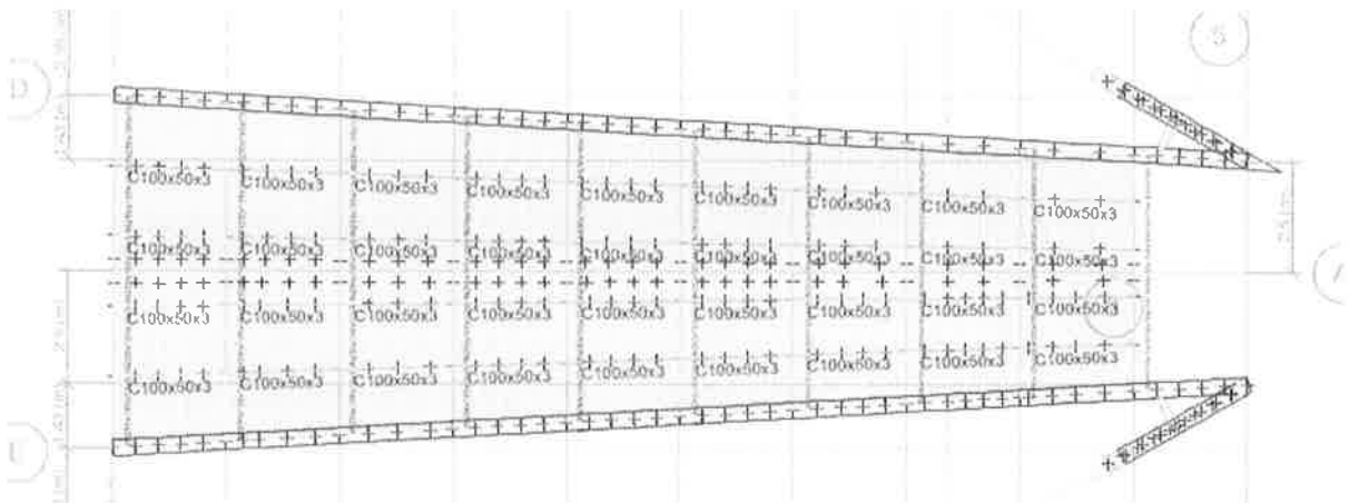
Ilustración – Estructura de techo propuesta, compuesta por vigas principales transversales IN 25 x 24,7 a 2,5 m aproximadamente y vigas secundarias longitudinales CA 10 x 4,95 a 1 m aproximadamente.
