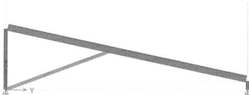
Ilustración – Refuerzo diagonal propuesto en los marcos de los ejes A, E, I, M, Q, U y X, compuesto por un perfil cajón 4 x 1,68 soldados en sus extremos. Ejes según planos de cálculo del edificio principal.
