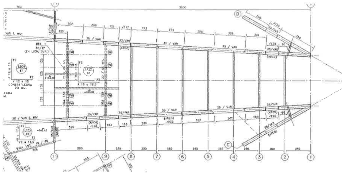
Ilustración – Plano de planta del sector de acceso al recinto, donde se dispondrá la estructura de techo a ejecutar.
