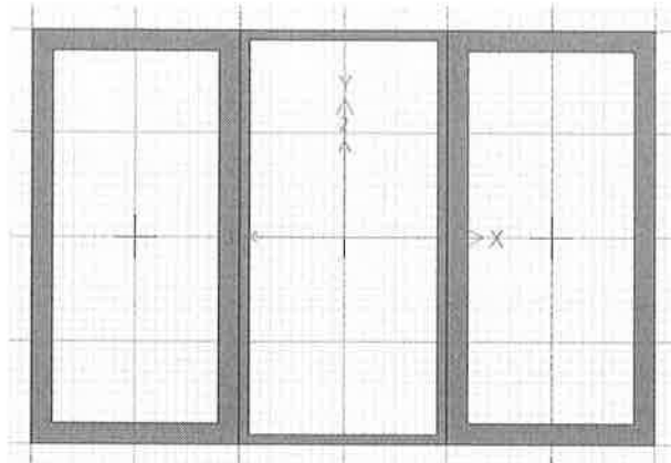
Ilustración – Refuerzo propuesto en los pilares, compuesto por un perfil cajón 4 x 0,89 existente y 2 perfiles cajón 4 x 1,68 soldados entre si.
