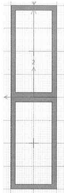
Ilustración – Refuerzo propuesto en vigas de los ejes A al X, reemplazando el perfil existente por dos perfiles cajón 4 x 1,68 soldados entre si. Ejes según planos de cálculo del edificio principal.
