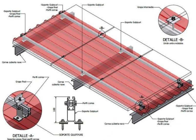
Ilustración 11 - Estructura tipo paralelo a cubierta en techo inclinado
